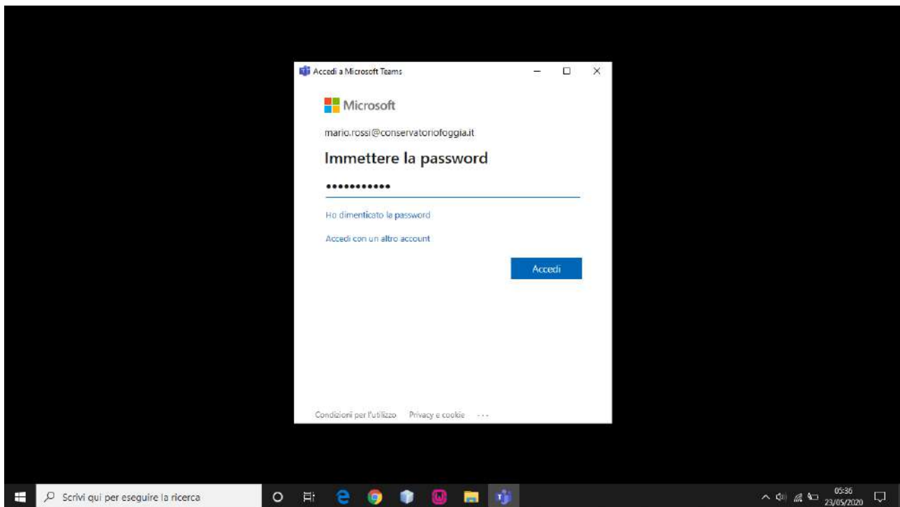
Figura 4 - Inserimento password
