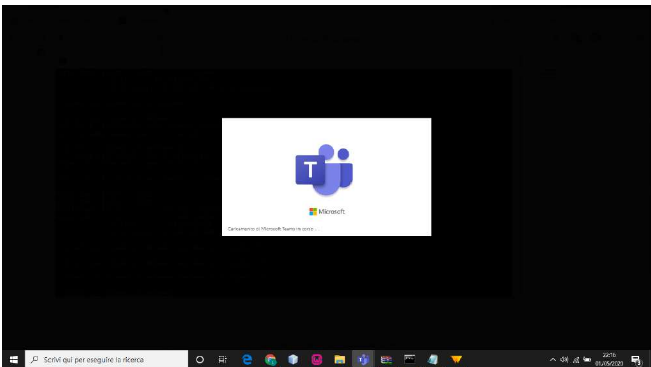
Figura 1 - Avvio dell'applicazione
