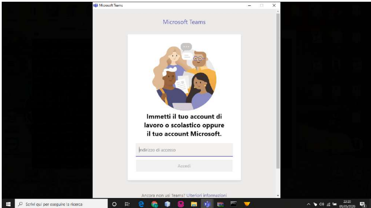
Figura 2 - Autenticazione
